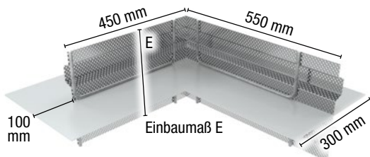
FUGENBLECH Abschalelemente Eck-Profil verzahnt – Typ S
