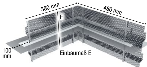
DICHTBLECH ABS Eck-Profil verzahnt – Typ S
