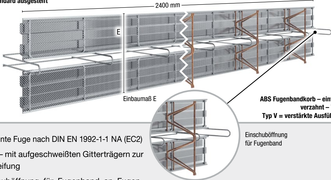
ABS Fugenbandkorb – einteilig, verzahnt – Typ S Typ S = Standard ausgesteift
