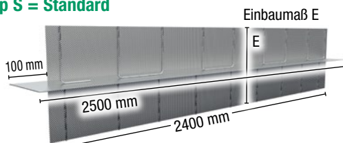
FUGENBLECH Abschalelemente rau – Typ S
