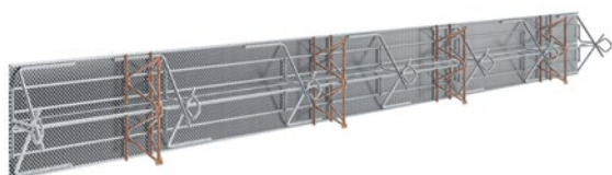
ABS Dichtblechkorb rau – Typ V Typ V = verstärkte Ausführung
