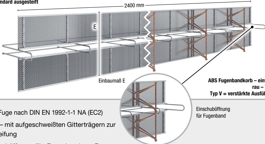
ABS Fugenbandkorb – einteilig, rau – Typ S Typ S = Standard ausgesteift
