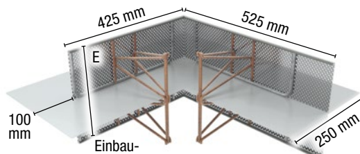
FUGENBLECH Abschalelemente Eck-Profil rau – Typ V
